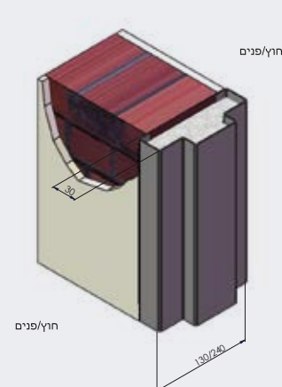
משקוף בניה סימטרי
