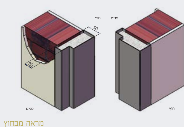
משקוף בניה אסימטרי סטנדרט קנט פנימי 30 מ"מ, קנט חיצוני 50 מ"מ
