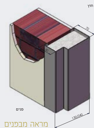
משקוף בניה אסימטרי קנט פנימי 50 מ"מ, קנט חיצוני 70 מ"מ
