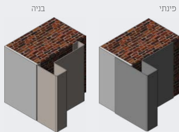
משקופי קו אפס
